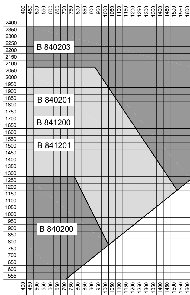
Flügelgrößendiagramm bezogen auf die Profilgeometrie Sash size diagram based on the profile geometry
